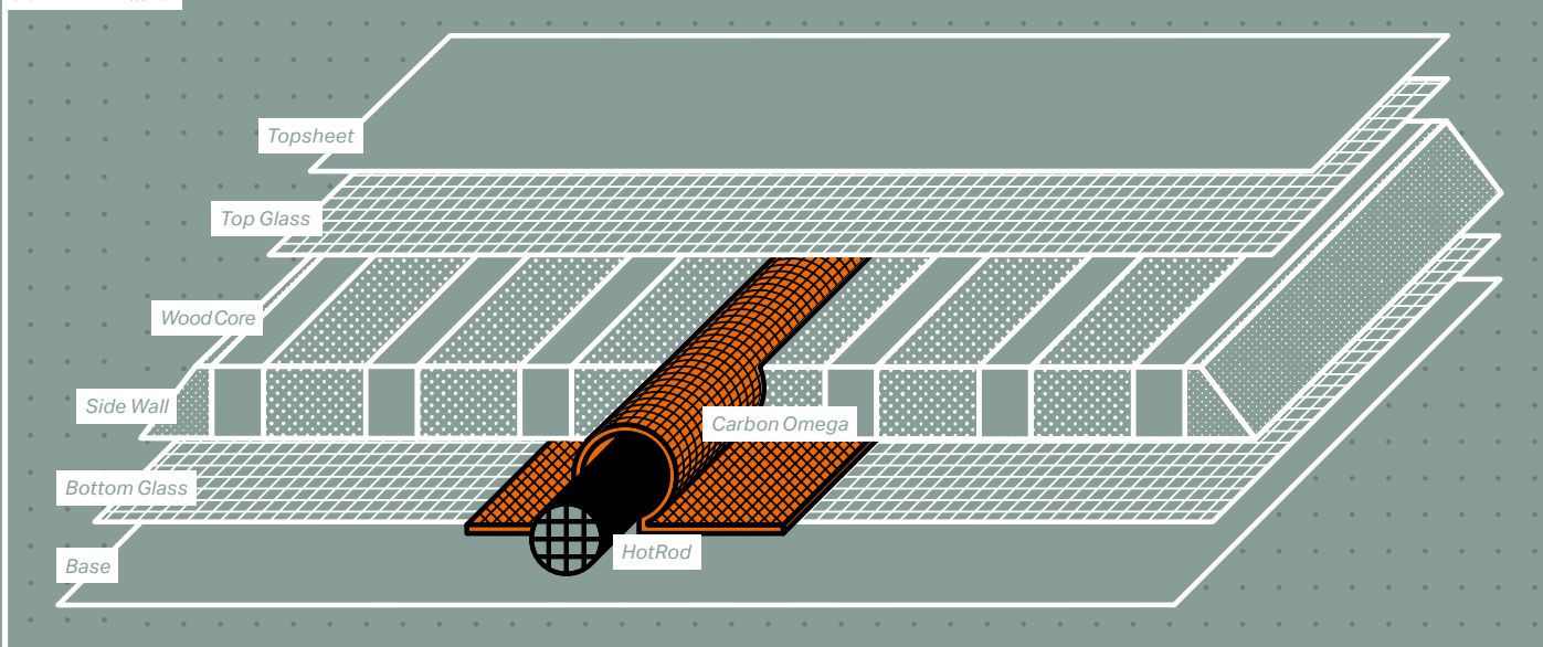
図1. ボード構造
