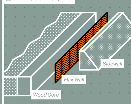
図3. フラックス・ウォール
