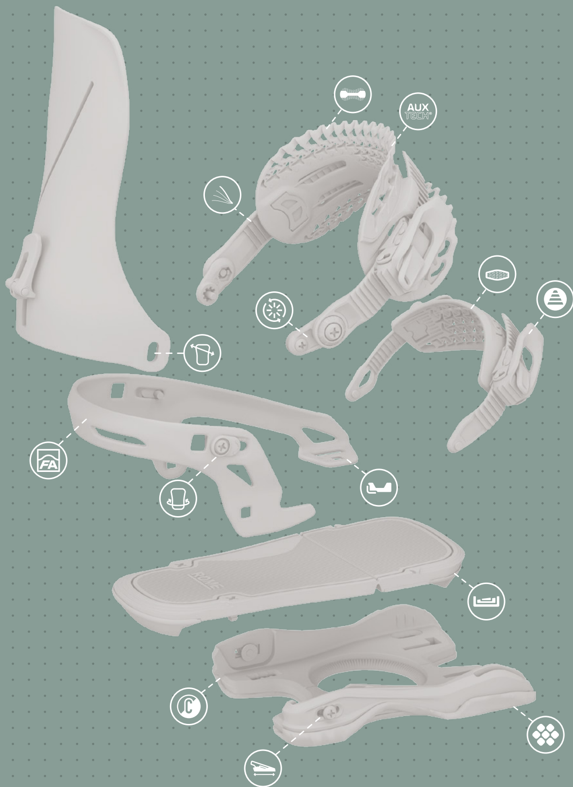
図1. バインディング分解図
