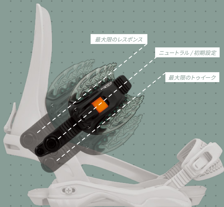
図3. ピボット・マウント
